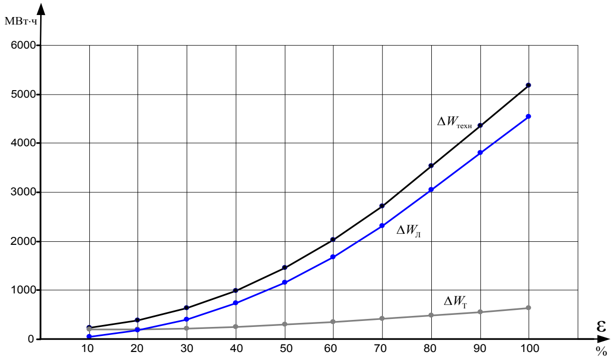
Рис. 1. Динамика изменения составляющих технических потерь ЭЭ (а – в процентах, б – в мегаваттчасах)
