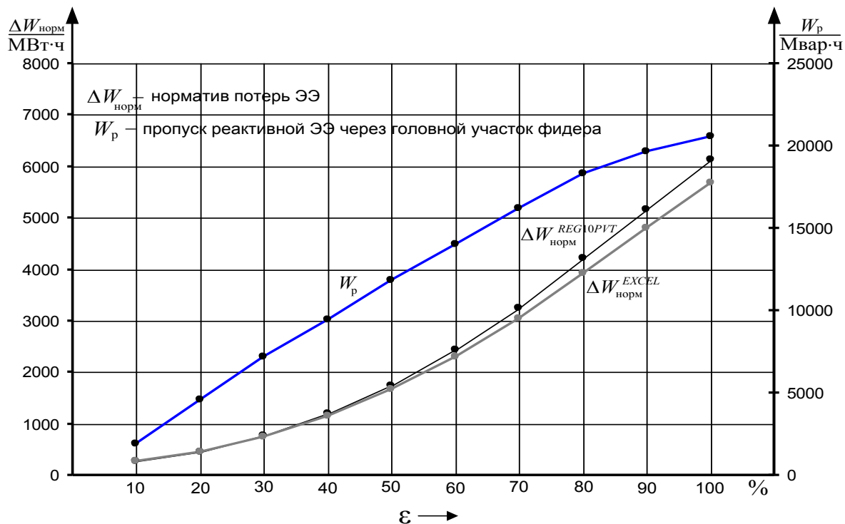
Рис. 3. Динамика изменения нормативов потерь ЭЭ
