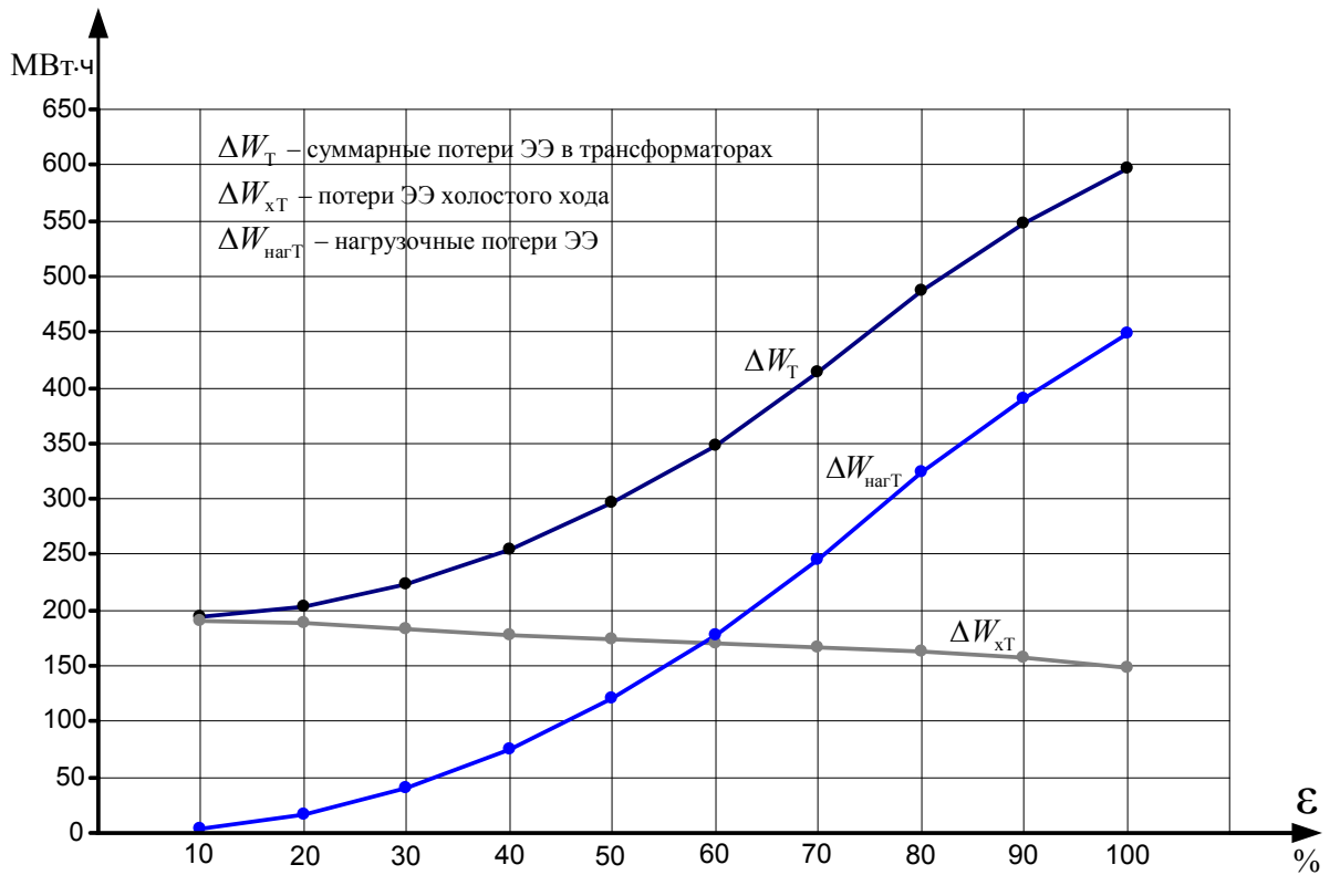
Рис. 2. Динамика изменения составляющих потерь ЭЭ в трансформаторах
