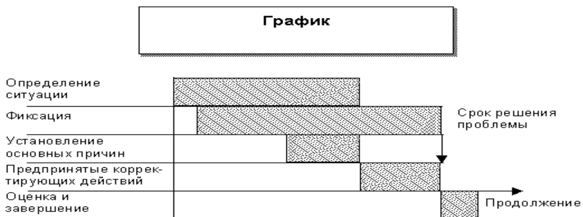
Рисунок 2 – График Ганта
