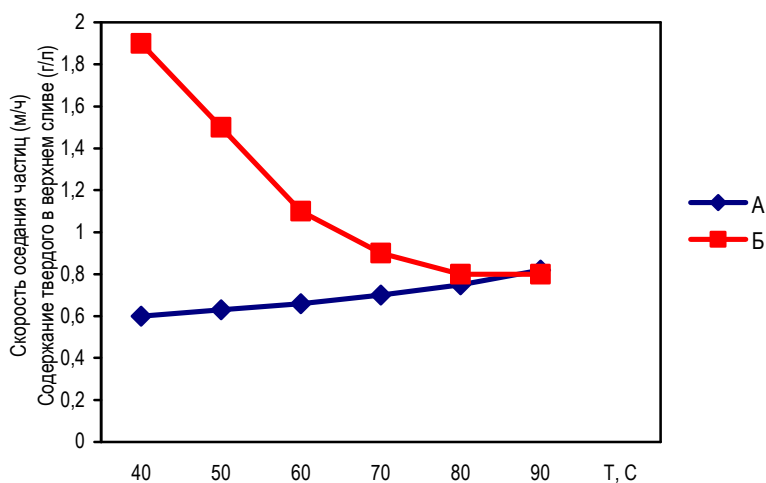
Рисунок 2. График зависимости: А – скорости оседания частиц (м/ч) и Б – содержания твердого в верхнем сливе (г/л) от температуры (флокулянт Zetag 32 (0,1%) в количестве 250 г/т твердого в пульпе).
