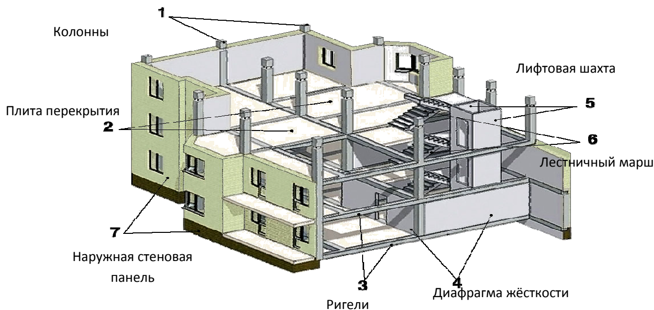
Рис. 1 Основные элементы сборно-монолитного каркаса, изготавливаемые на предприятии ООО "Монолитресурс"
