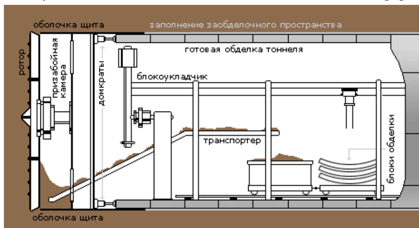
Рис. 1. Механизированный тоннелепроходческий комплекс со свободной призабойной камерой
