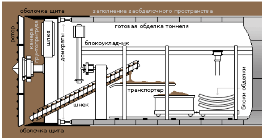
Рис. 2. Механизированный тоннелепроходческий комплекс с грунтопригрузом забоя
