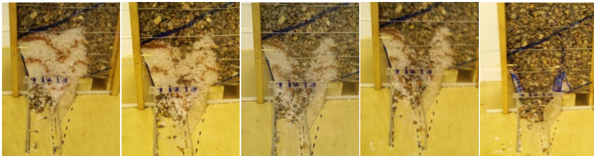
Рис.2 Процессы истечения материала, формирование зон потерь и разубоживания
