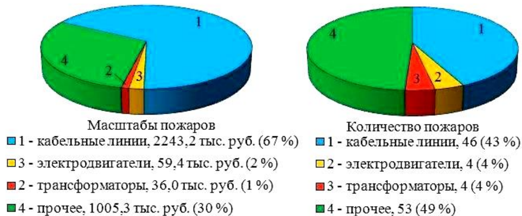
Рисунок 1 – Пожары, возникшие по электротехническим причинам, на предприятиях нефтегазовой отрасли на территории Российской Федерации (данные ВНИИПО за период с 1997 г. по 2009 г.)
