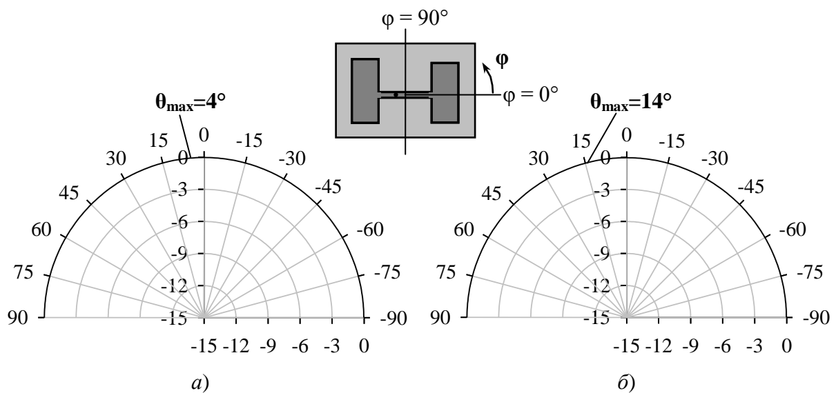
Рис. 3. Результаты расчета амплитудных диаграмм направленности на частоте f_I = 8.99 \text{ ГГц} в плоскостях \varphi = 0^\circ (а) и \varphi = 90^\circ (б)
