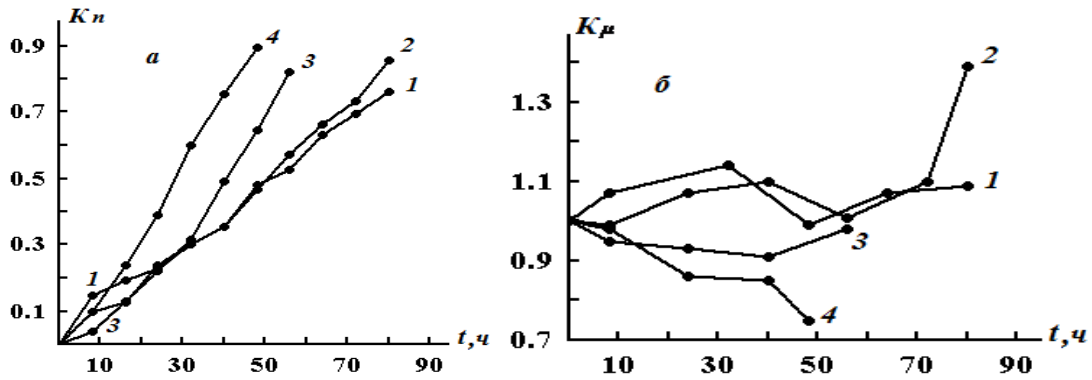
Рис. 1. Зависимость коэффициентов поглощения светового потока K_n (а) и относительной вязкости K_\mu (б) от времени окисления минеральных моторных масел: 1 – М10-Г 2К ; 2 – М8-Г 2 ; 3 – Лукойл стандарт 10w-40 SF/CC; 4 - Utech navigator 15w-40 S6/CD
