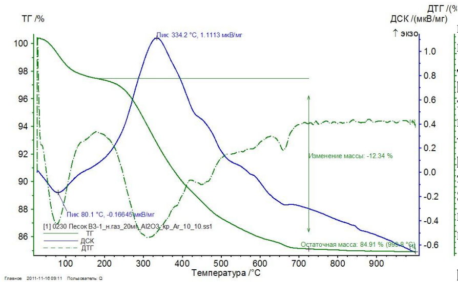
Рис.2 – термограмма отходов сжигания
