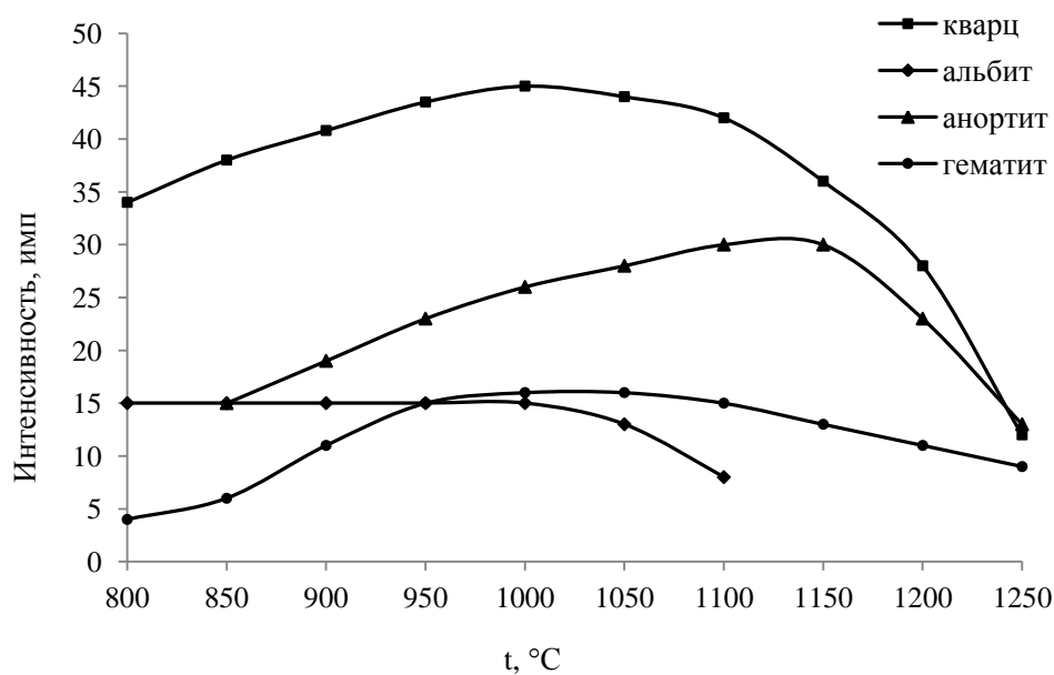
Рис. 4. График изменения минералов в зависимости от температуры обжига для состава Компановская глина 85% + кек красный 15%
