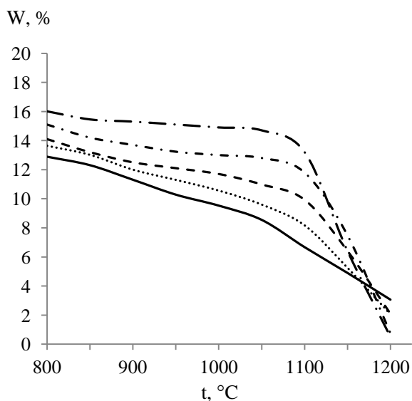
Рис. 2. Зависимость водопоглощения образцов от температуры обжига.
