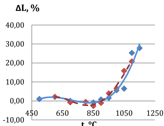
Рис. 3. Кривая зависимости огневой усадки от температуры обжига
