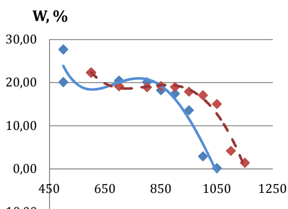
Рис. 4. Кривая зависимости водопоглощения от температуры обжига
