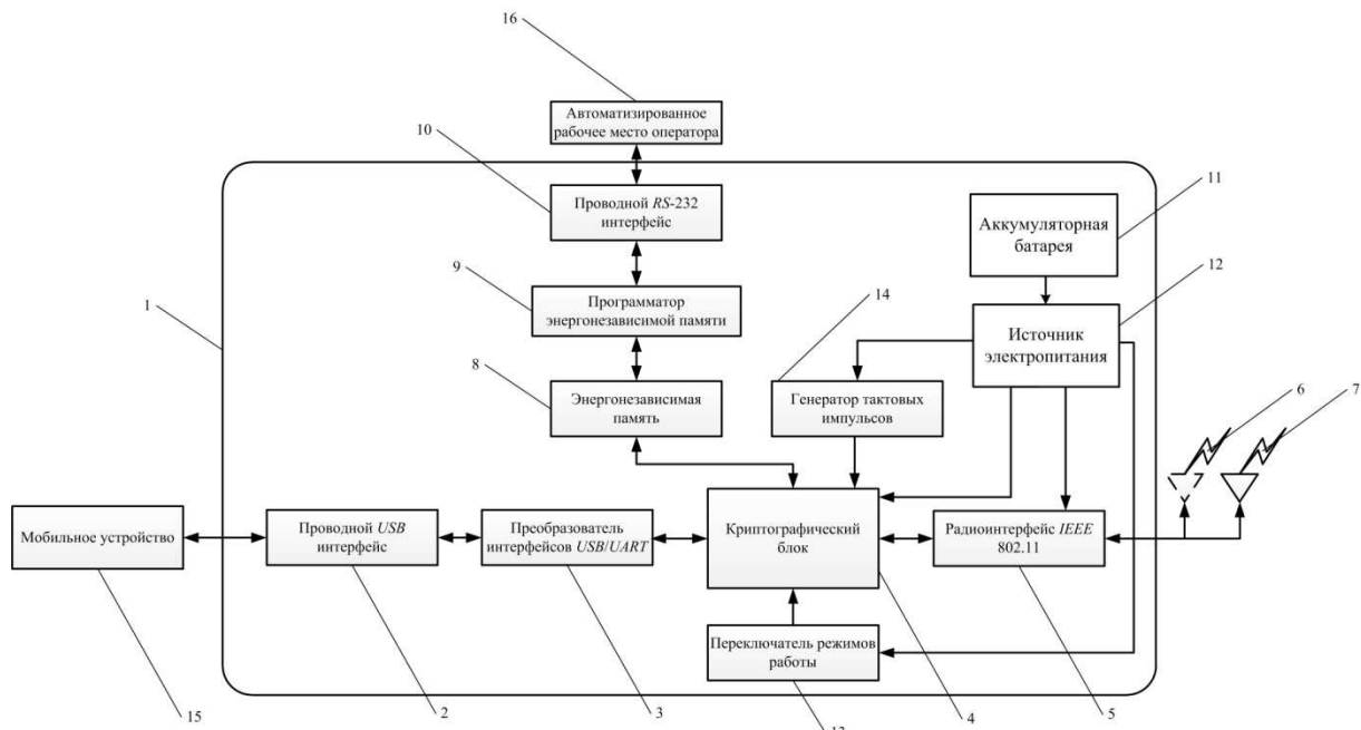
Рис. 1. Структурная схема устройства обеспечения защищенной передачи данных
