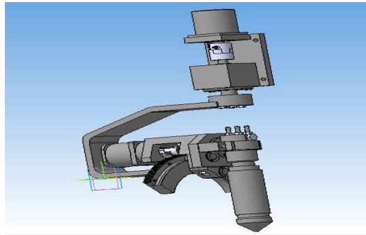
Рисунок 4 – Модель наклонного механизма с круговым сектором
