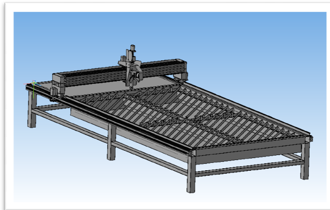
Рисунок 5 – Общая сборка станка
