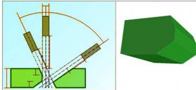
Рисунок 2 – Подготовка кромок под сварку
