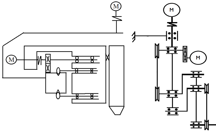
Рисунок 3 – Схемы наклонных с круговым сектором и рычажного механизмов
