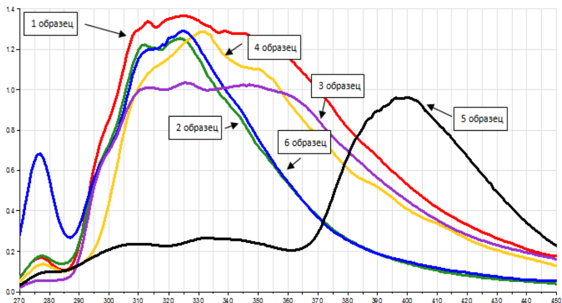
Рисунок 3 - Сводный график спектров флуоресценции образцов, при температуре 300 °С
