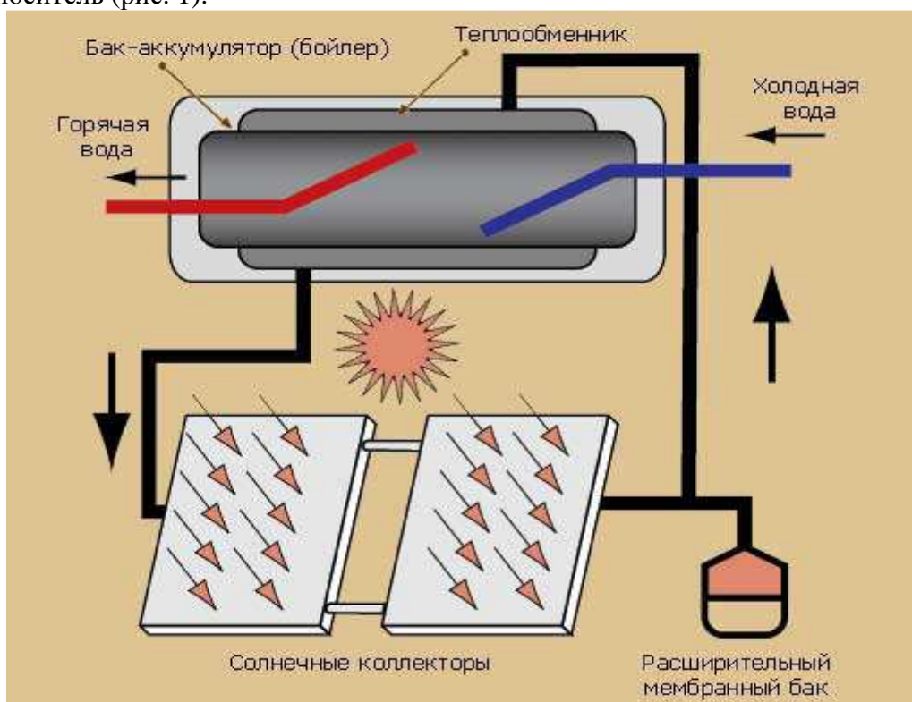
Рисунок 1- Принципиальная схема двухконтурного термосифонного солнечного водонагревателя
