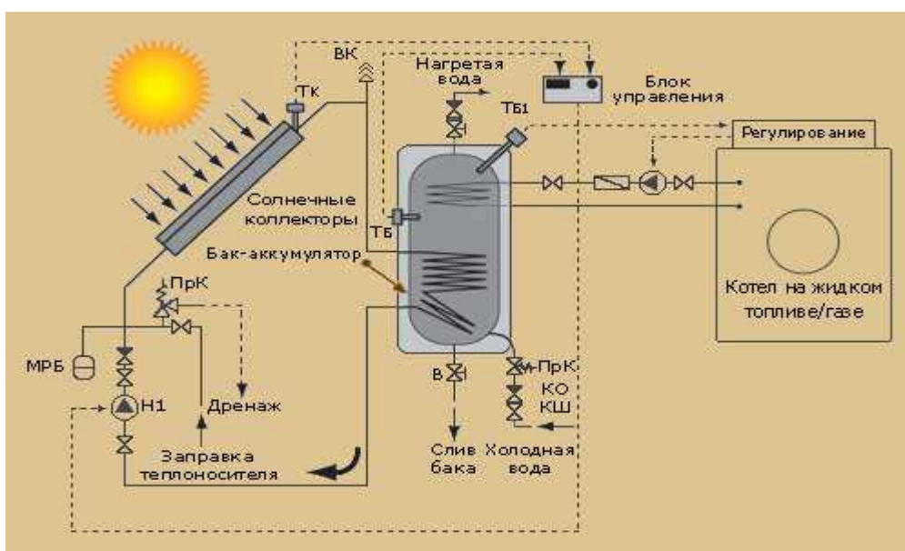
Рисунок 2- Принципиальная схема системы солнечного водоснабжения
