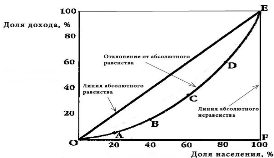
Рис. 1 Кривая Лоренца
