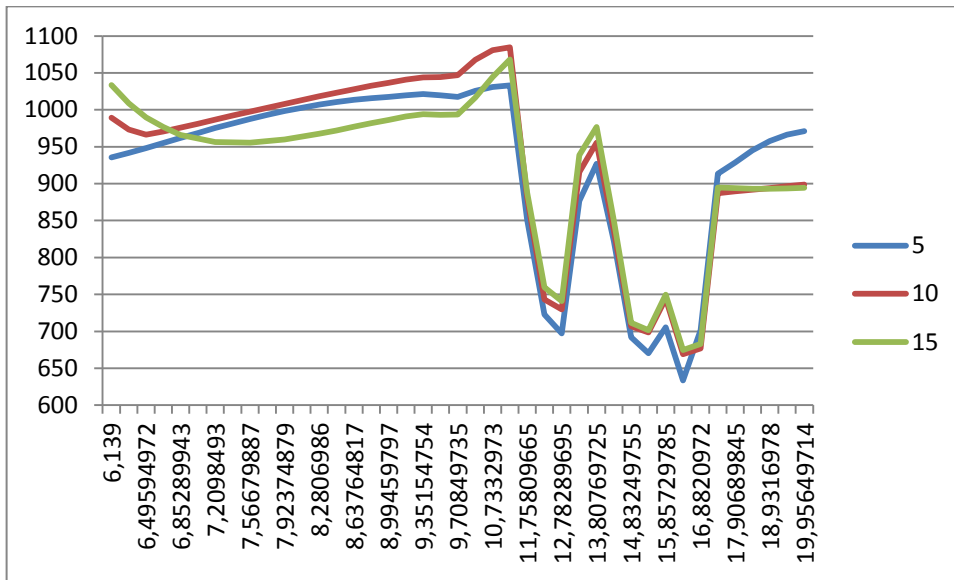
Рис. 4. График зависимости температуры приэкранного слоя от высоты топки при различных углах наклона горелок нижнего яруса.
