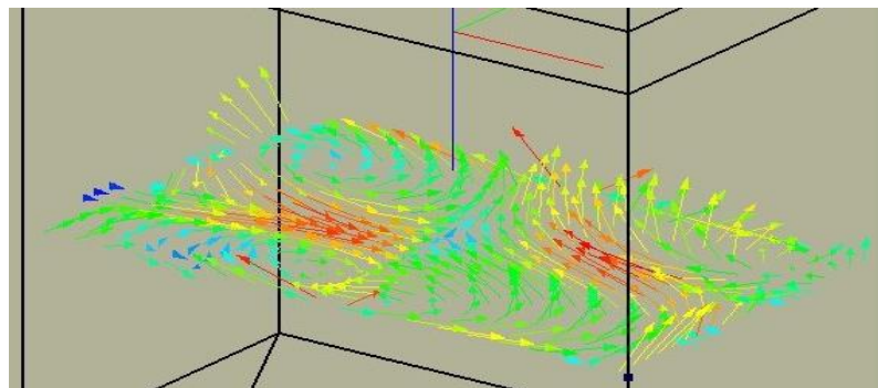
Рисунок 3 – Поле скоростей
