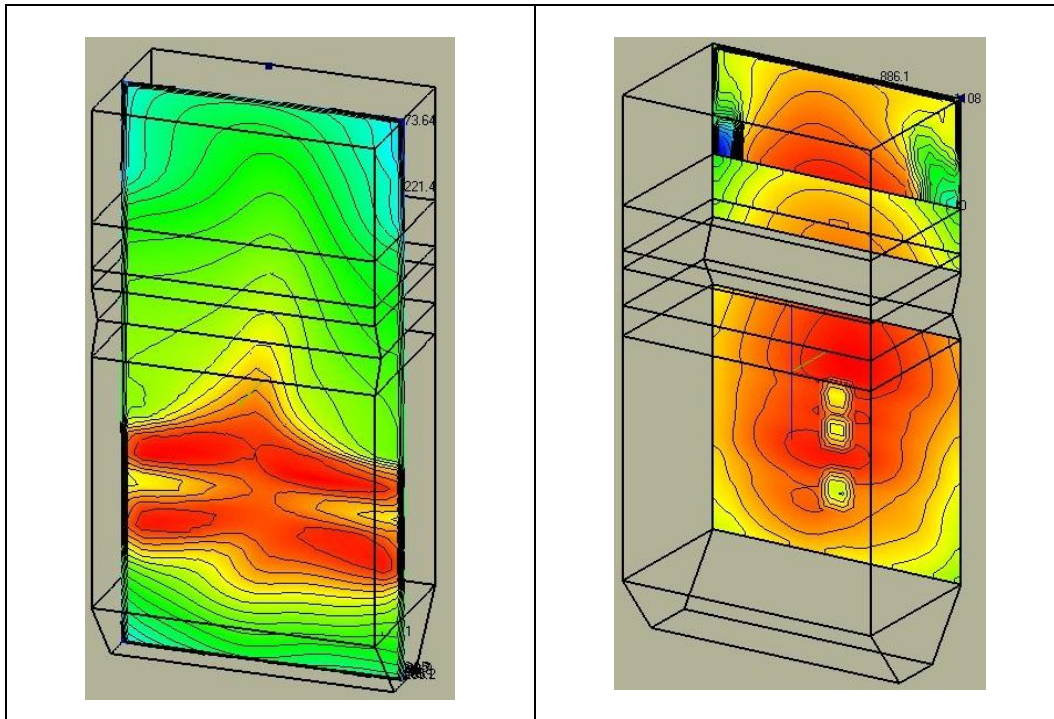
Рисунок 2 – Поле температур
